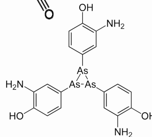
Salvarsan
